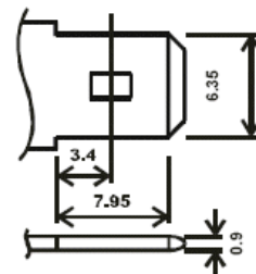
SR-pole
